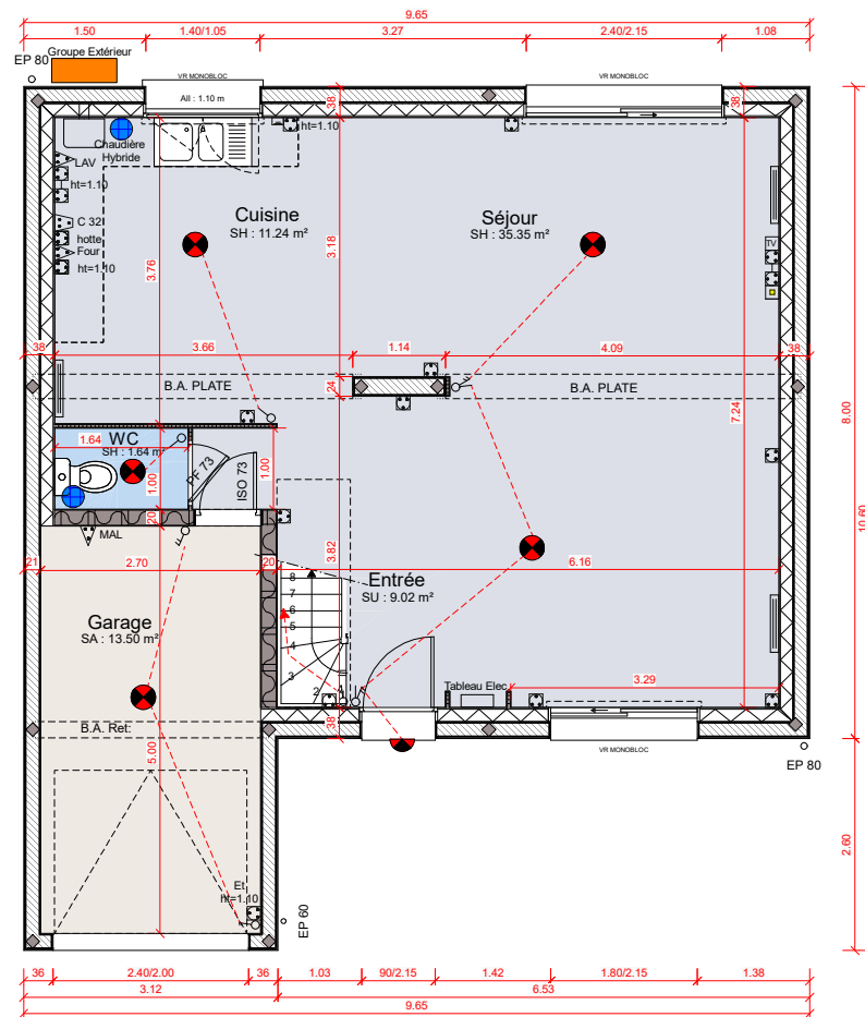
REZ-DE-CHAUSSEE
