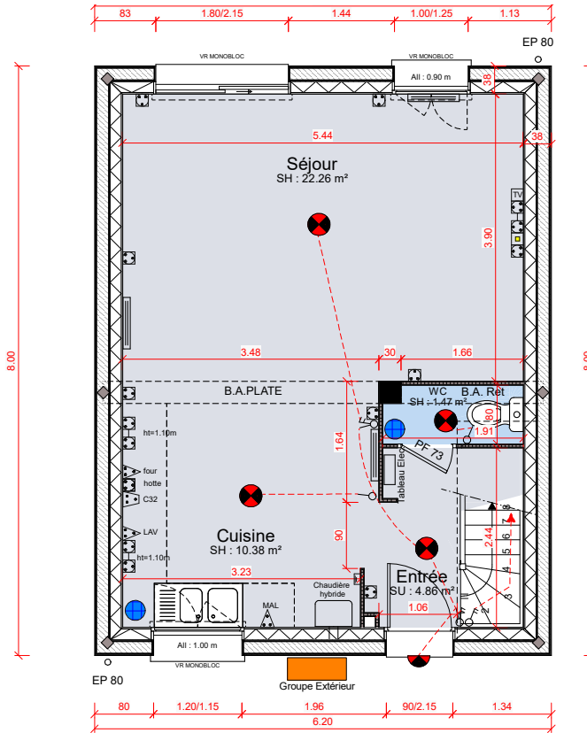
REZ-DE-CHAUSSEE
