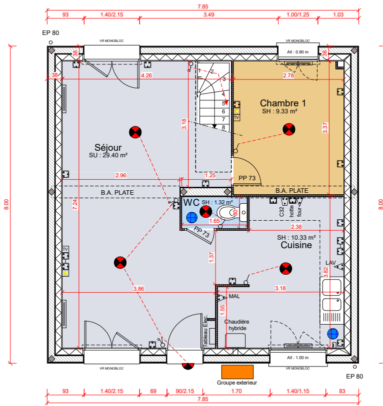
REZ-DE-CHAUSSEE
