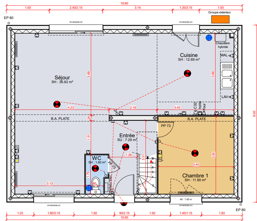
REZ-DE -CHAUSSEE
