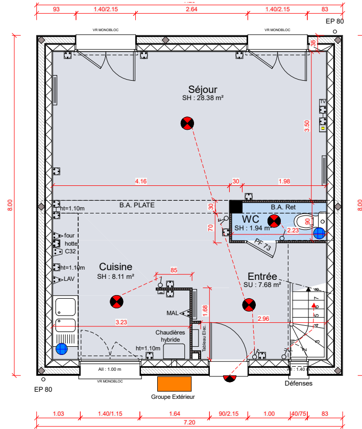
REZ-DE-CHAUSSEE
