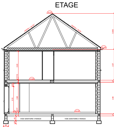
Coupe
