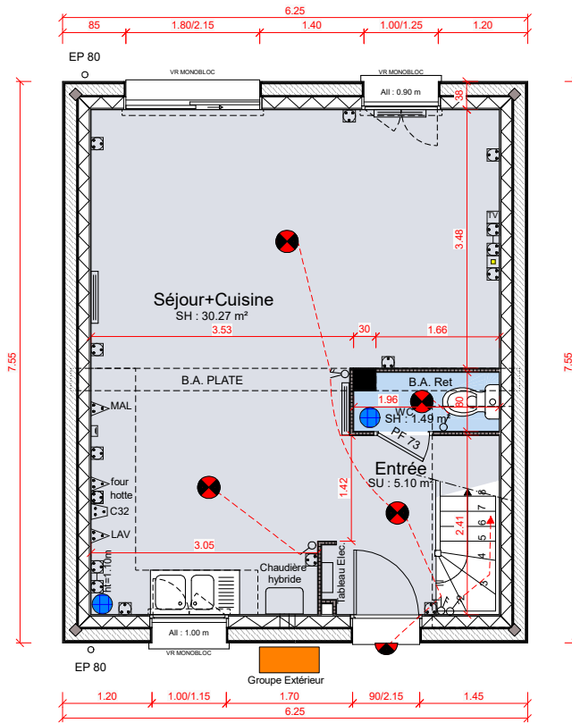
REZ-DE CHAUSSEE
