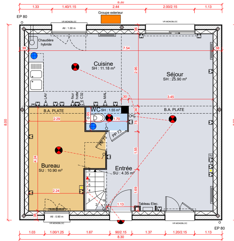
REZ-DE-CHAUSSEE
